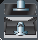
埋め込み構造スパイクピン断面イメージ図 WDシリーズは、「カシメタイプ」のピンを「埋め込みタイプ」にすることで、より抜けにくい構造となっているのが特徴です。
